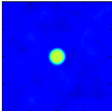
TrapezoidDisk2DKernel
